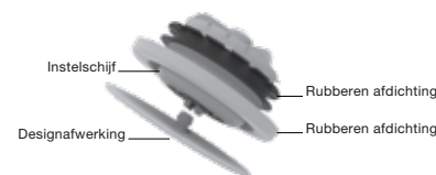
ComfoValve Luna E, explosietekening
