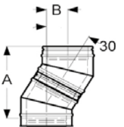
Afb. Bocht 45°
