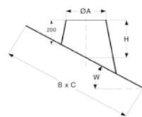
Dakdoorvoer 36° - 45° (met loodslab)
