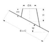
Dakdoorvoer 16° - 25° (met loodslab)
