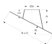
Dakdoorvoer 26° - 35° (met loodslab)
