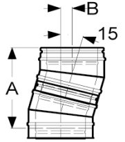
Afb. Bocht 30°
